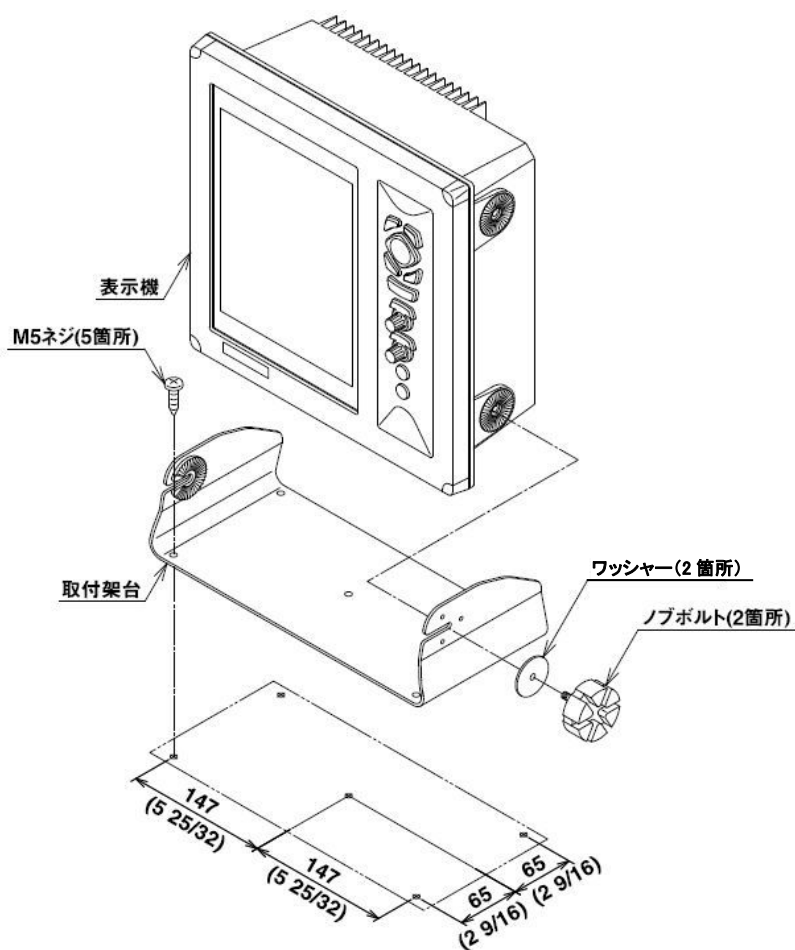
図 5.2 卓上取付図
