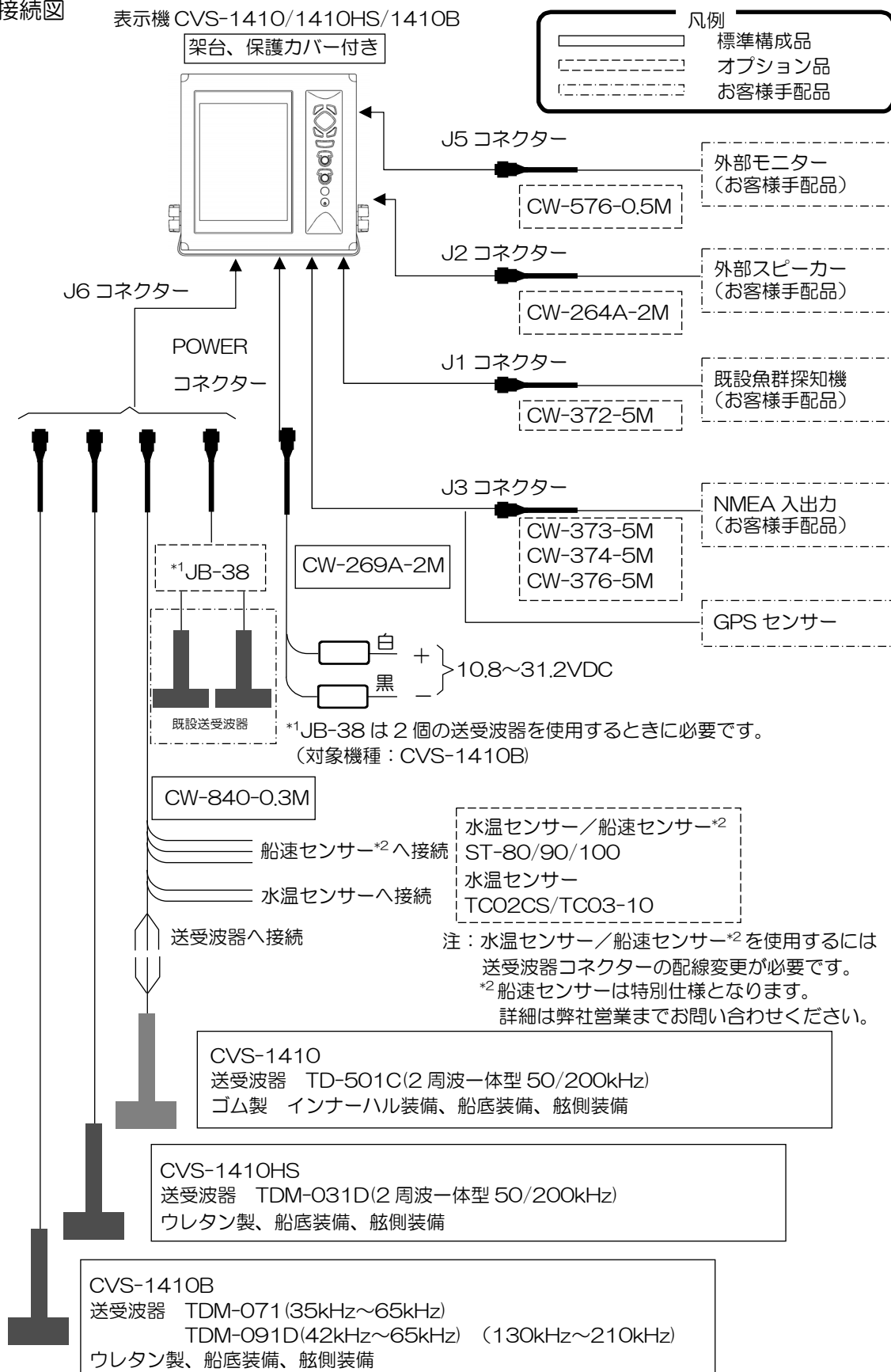
接続図
