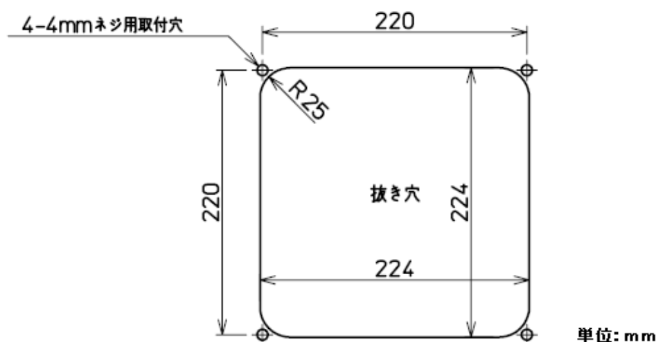
図 5.5 フラッシュマウント取り付け穴加工図
