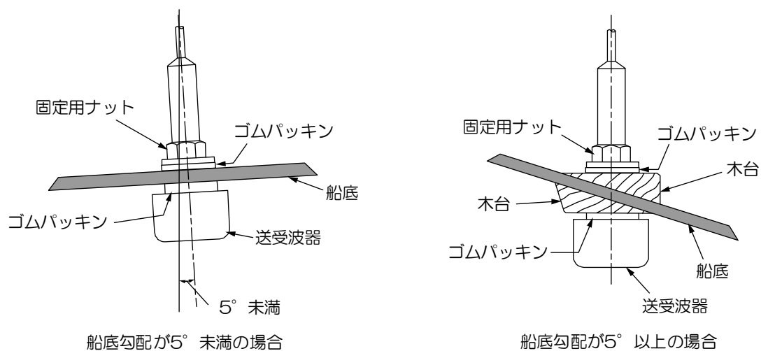
図 5.8 スルーハル取り付け図
