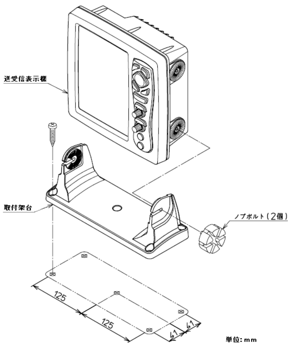
図 5.2 卓上取付図
