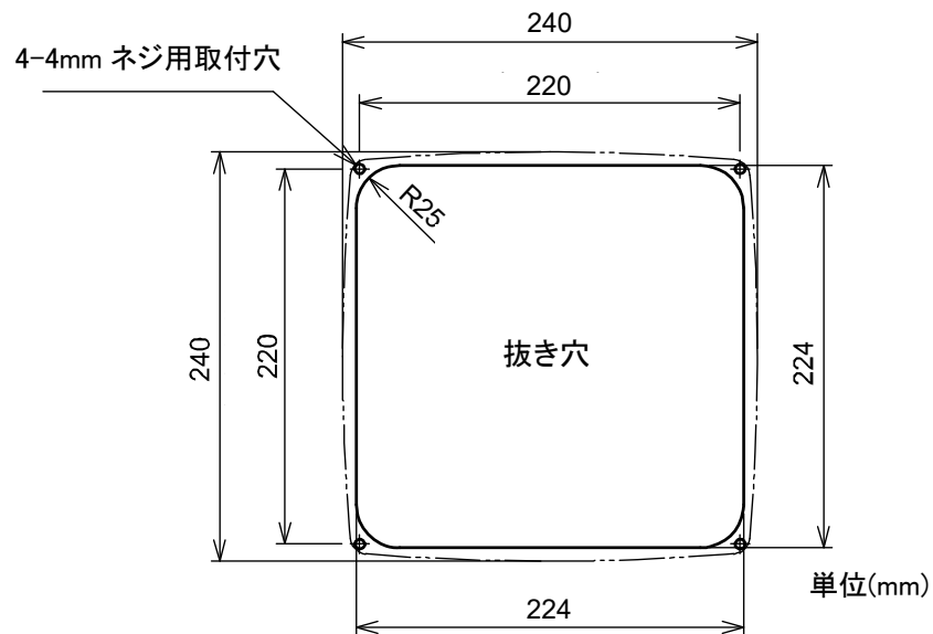
フラッシュマウント設置寸法図
