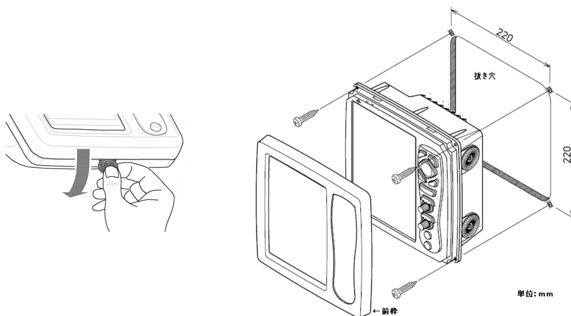
図 5.4 フラッシュマウント取付図
