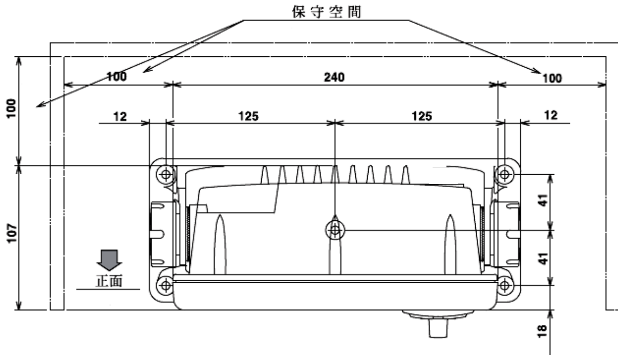
卓上設置寸法図
