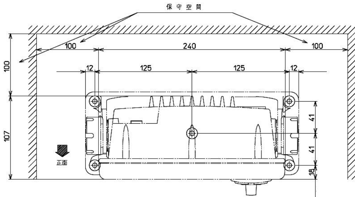
図 5.3 保守空間
