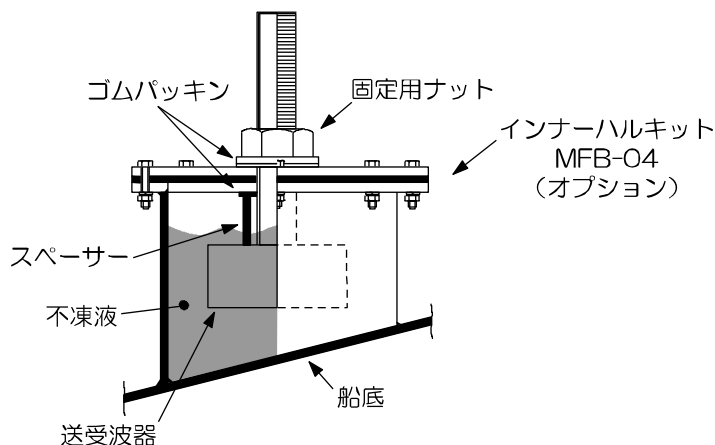
図 5.7 インナーハル取り付け図
