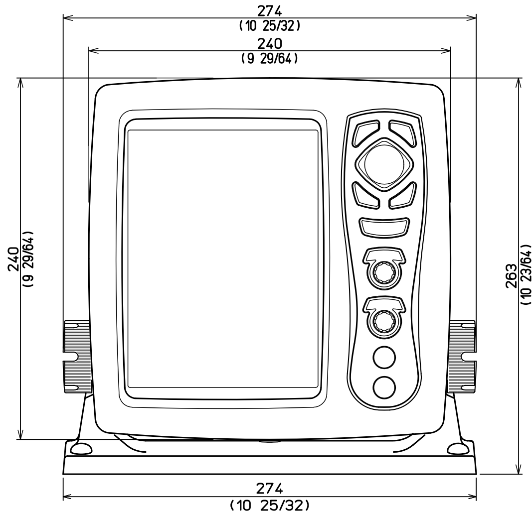
Front view 正面図
