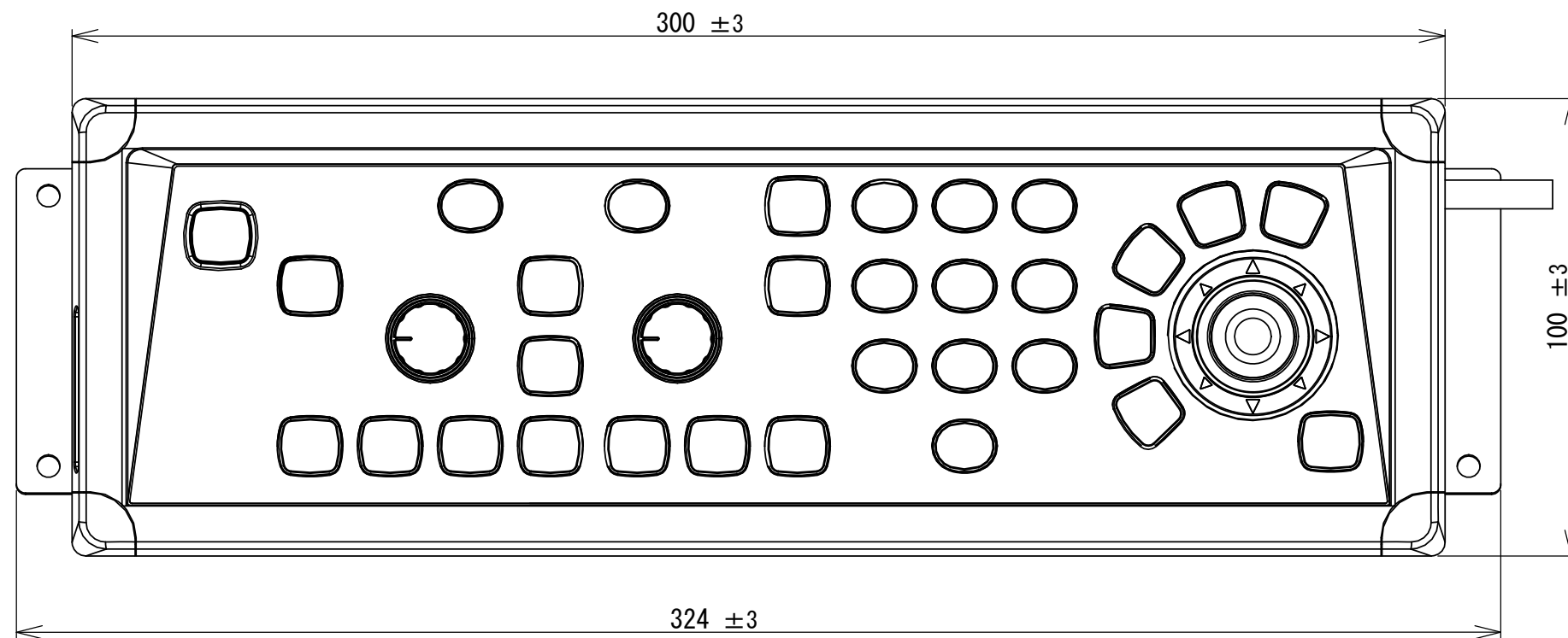
Front view 正面図
