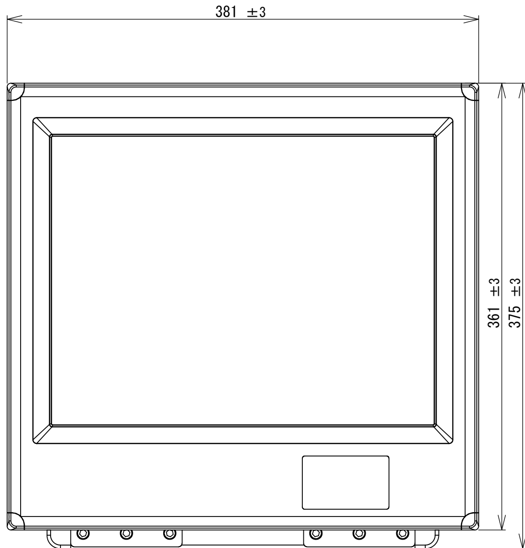
Front view 正面図
