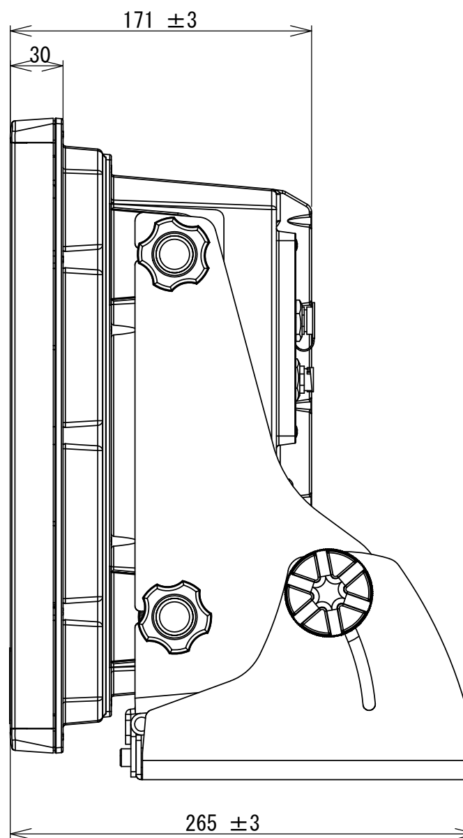
Side view 側面図
