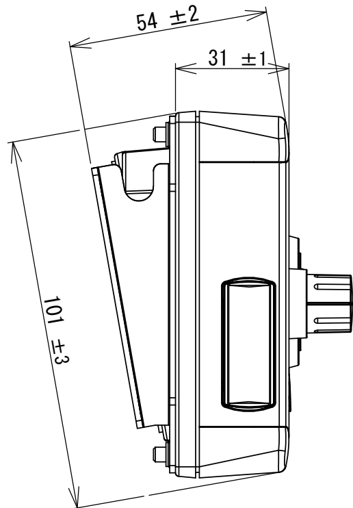
Side view 側面図
