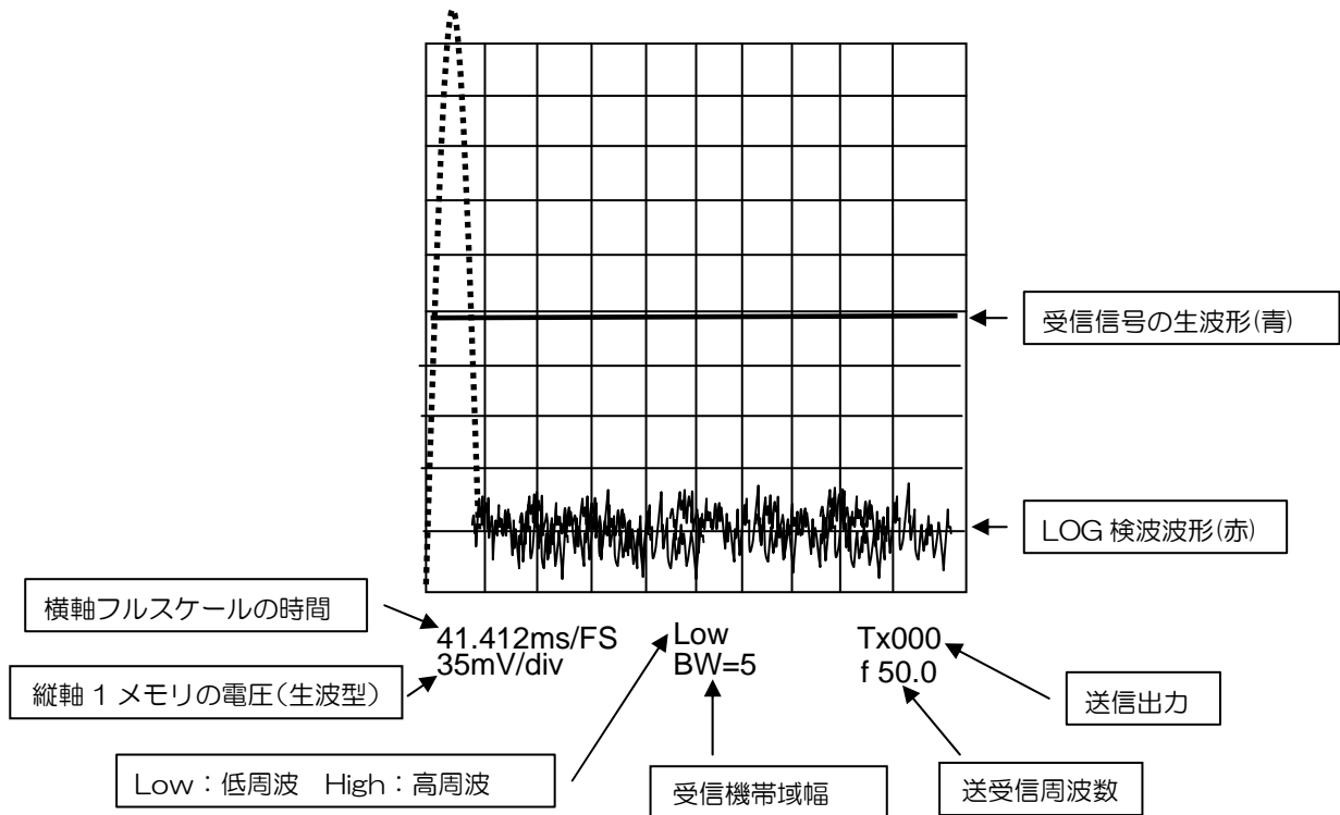
図 3.2 送信時のオシロスコープ画面
