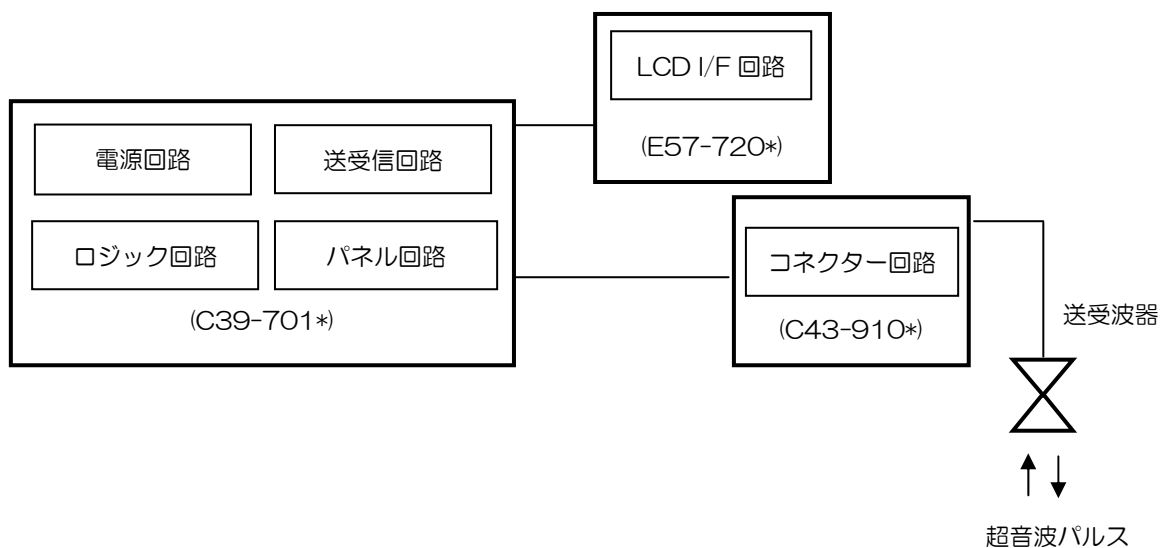
図 1.1 CVS-1410/1410HS/1410B/8410 回路構成図
